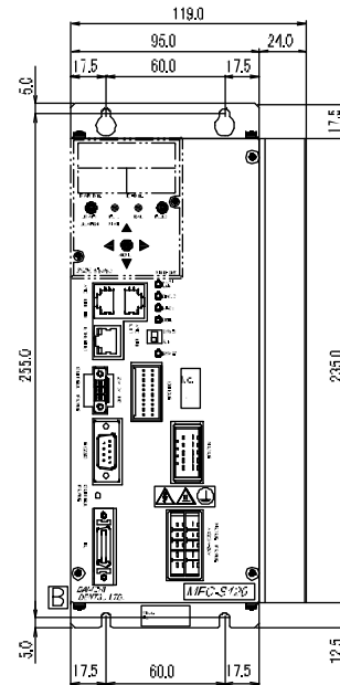
正面図(表示器付)
