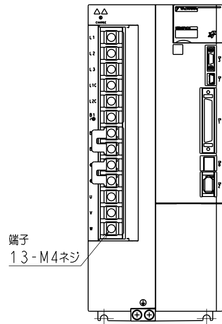
端子部詳細図
